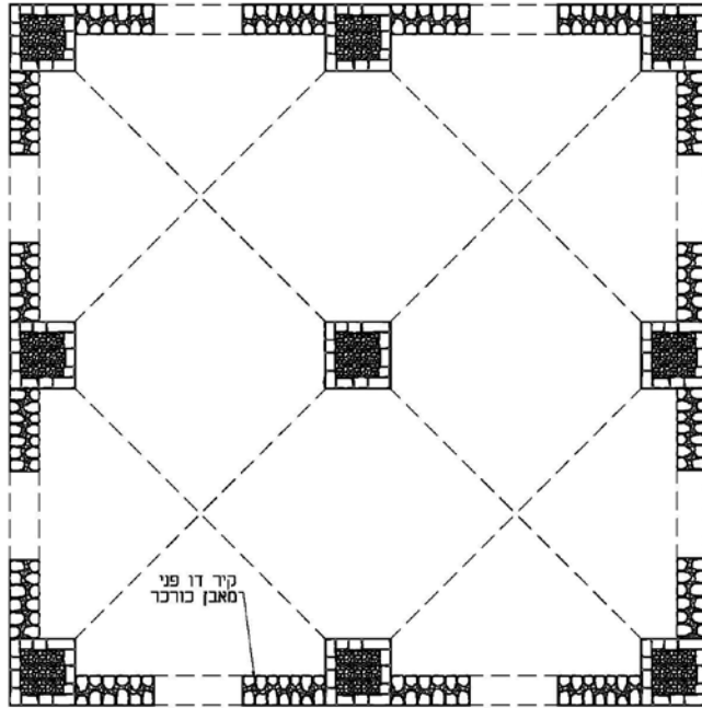
תכנית קומת קרקע חלופה ב- קיר קנ"מ 1:100
