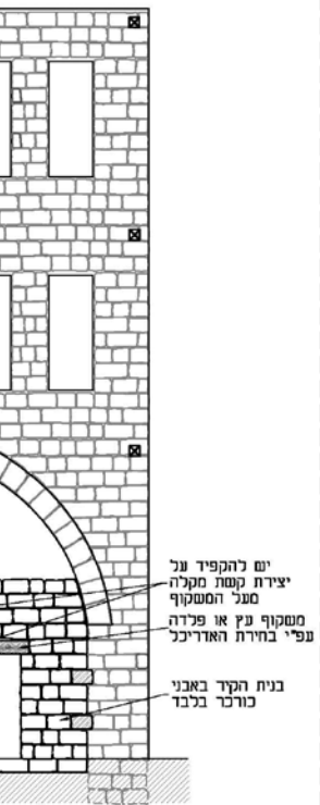
חזית - חלופה קנ"מ 1:100
