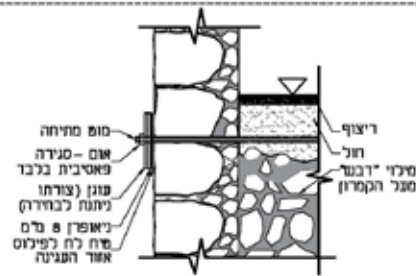
פרט עוגן מתחת לריצוף קנ"מ 1:20
