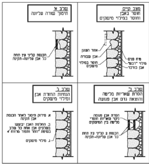
פרט טיפול באזור המיועד לעיגון קנ"מ 1:20
