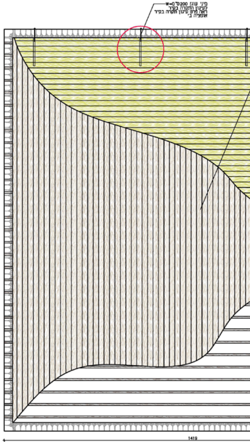
גית שכבות תקרת עץ קני"מ 1:50
