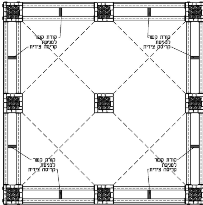
תכנית קומת קרקע חלופה א - קורות קנ"ח 1:100
