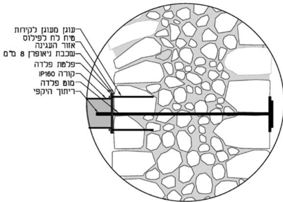
עיגון קורה לאומנה קנ"ח 1:20
