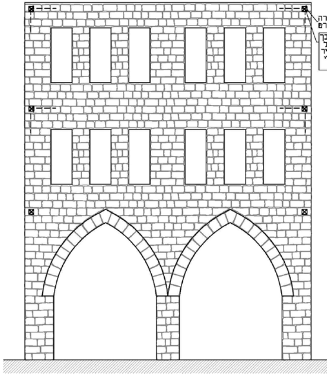
חבט עוגנים בחזית קנ"מ 1:100
