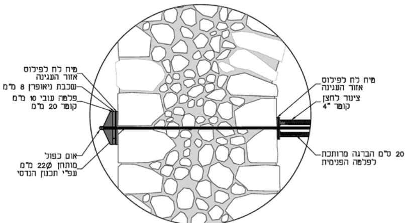
פרט מותחן לחצן קנ"ח 1:20
