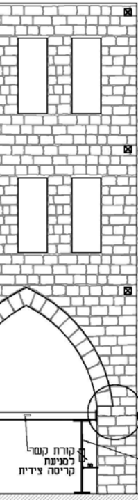
חזית - חלופה א' קנ"מ 1:100
