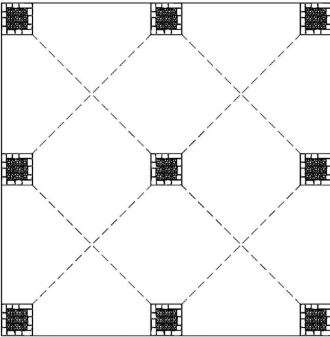
תכנית קומת קרקע מצב קיים קני"ח 1:100
