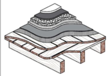
פרט שכבות תקרת עץ
