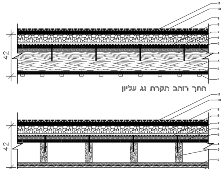
איור 11 | חתכים בתקרה עליונה, גג המבנה (נספח ג' 3)
