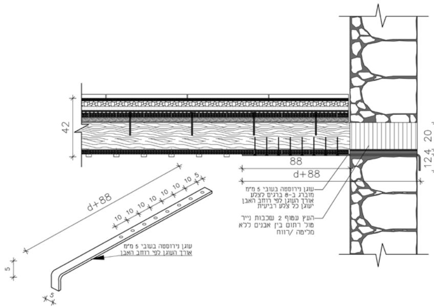
איור 9 | פרט עיגון תקרת עץ בקיר, חלופה א' (נספח ג' 4)
