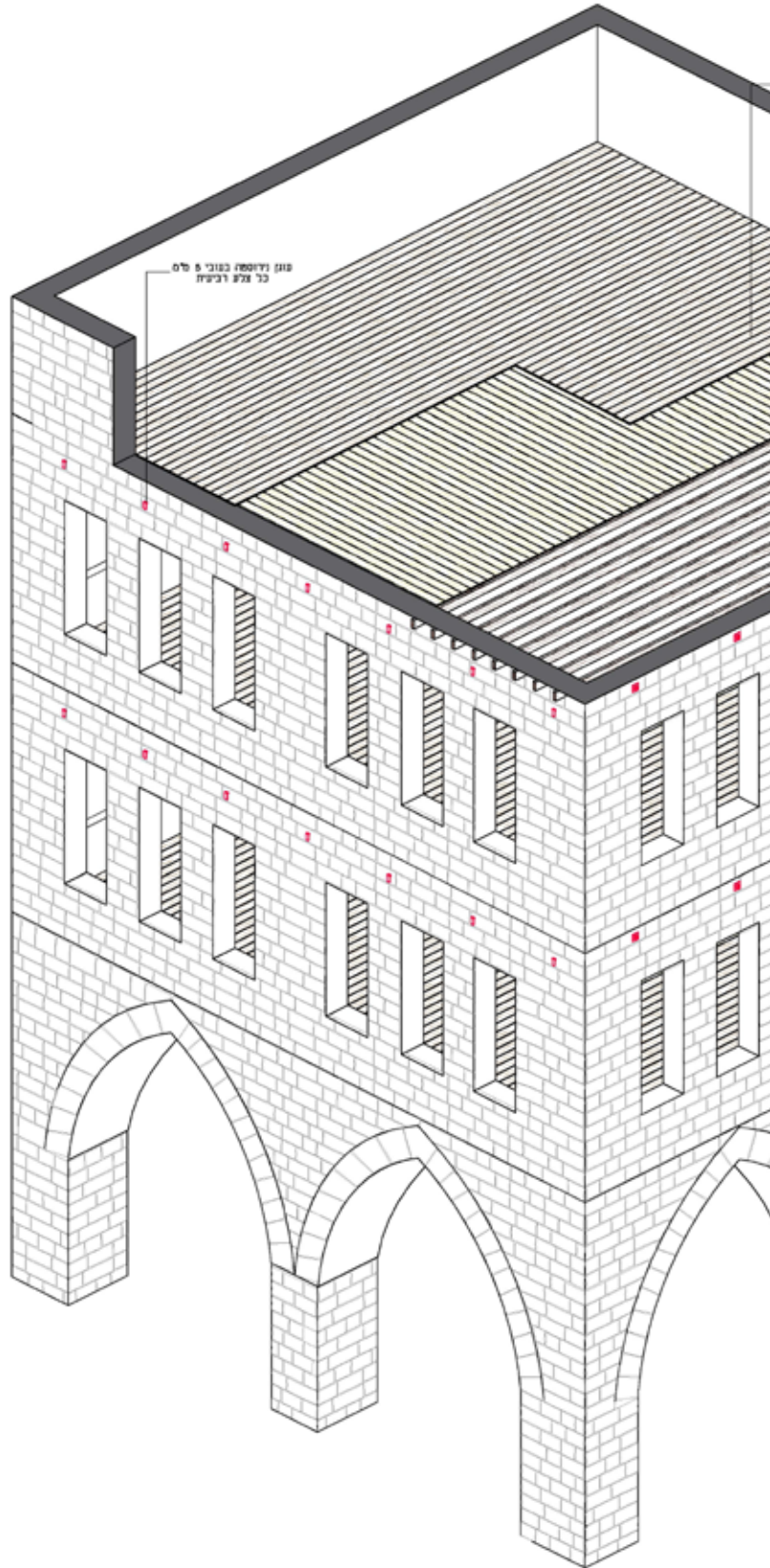
איזמעריה מבנה בעל תקרות עץ קנ"ח 1:50
