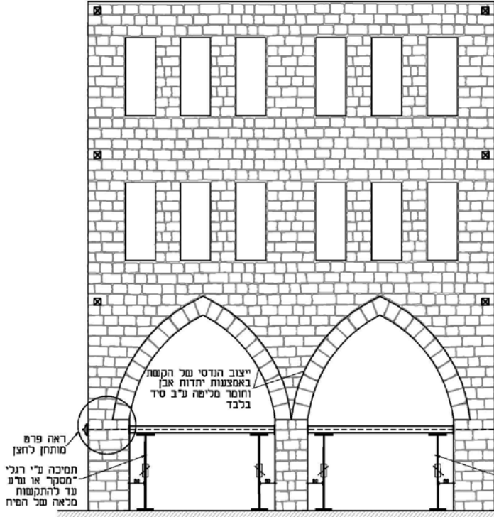
חזית - חלופה א2: מותחן להצן קנ"מ 1:100
