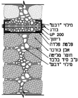
משקוף פלדה קנ"מ 1:20
