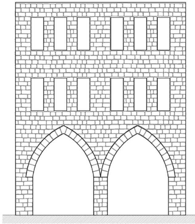
חזית מצב קיים קנ"מ 1:100
