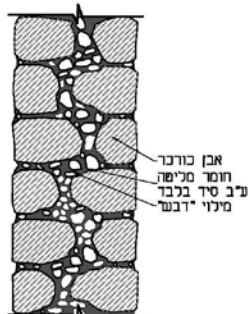
60 חתך קיר בשיטת ראש פתיון קנ"מ 1:20
